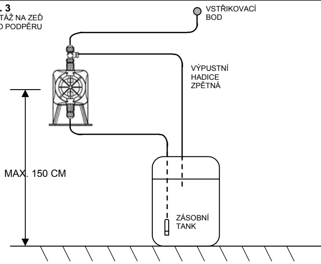
Obr. 4 MONTÁŽ SE ZATOPENÝM SÁNÍM
