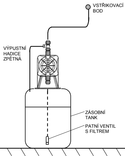
Obr. 5 MONTÁŽ NA ZÁSOBNÍ TANK
